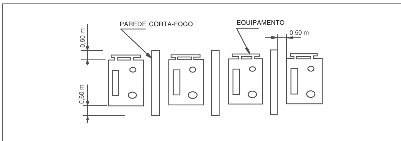
Figura 3: Separação por parede corta-fogo entre equipamentos
