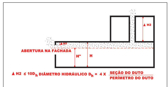
Figura 17: Diâmetro hidráulico
