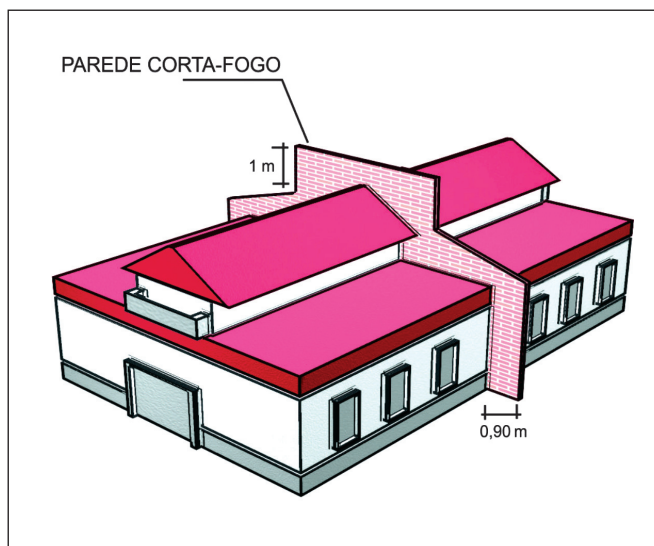
Figura 8: Parede corta-fogo
